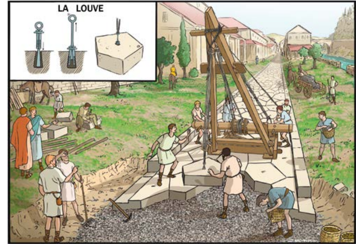
Dessin d'une scène présumée de construction de la voie romaine à l'aide d'une louve (dessin : J. Breteau conseillé par J.-M. Mignon)
